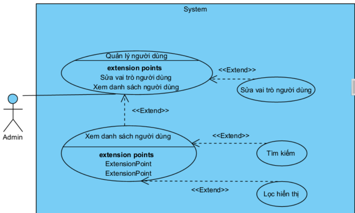
Hình 6 Use case quản lý người dùng
