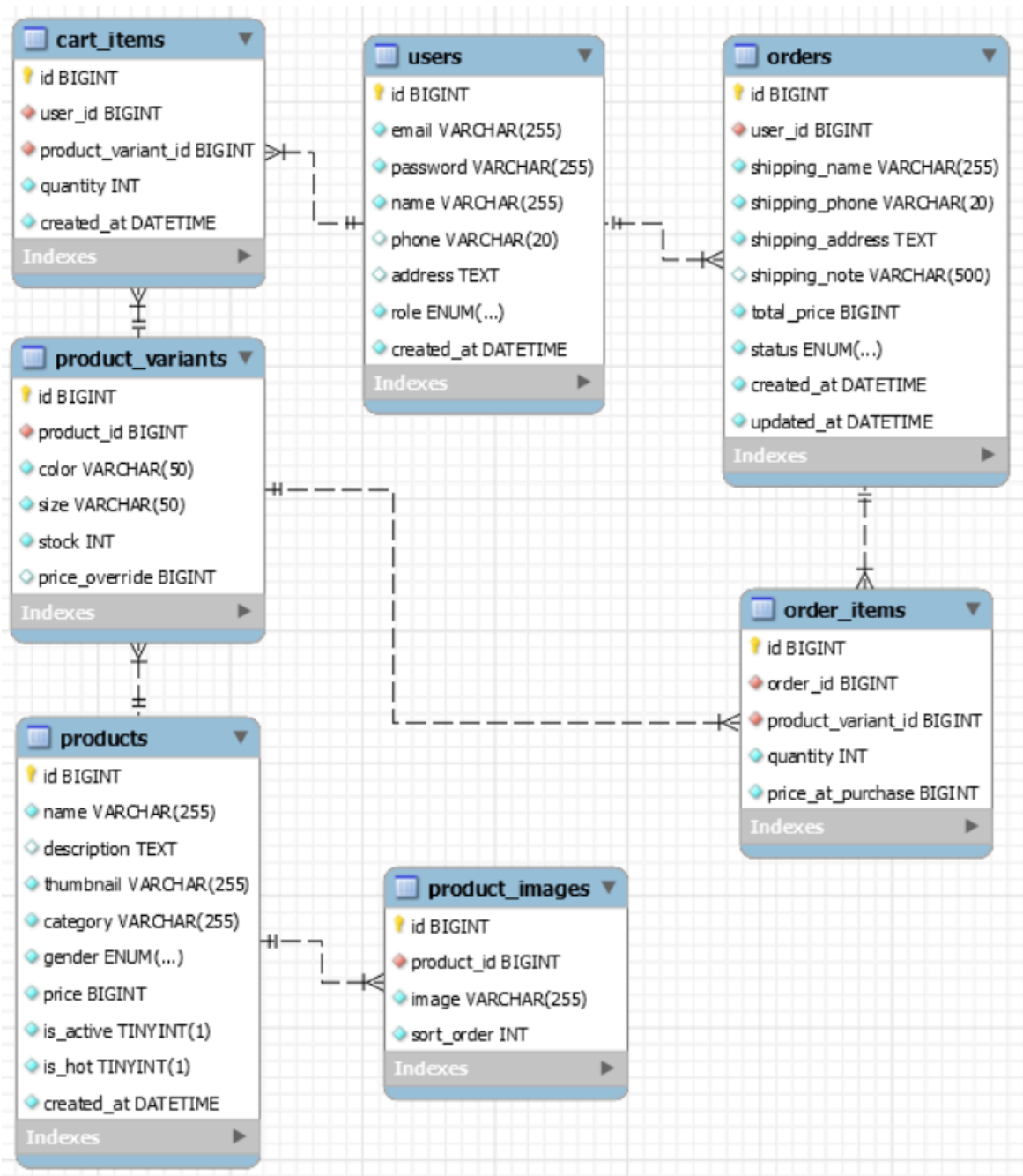
Hình 20 ERD
