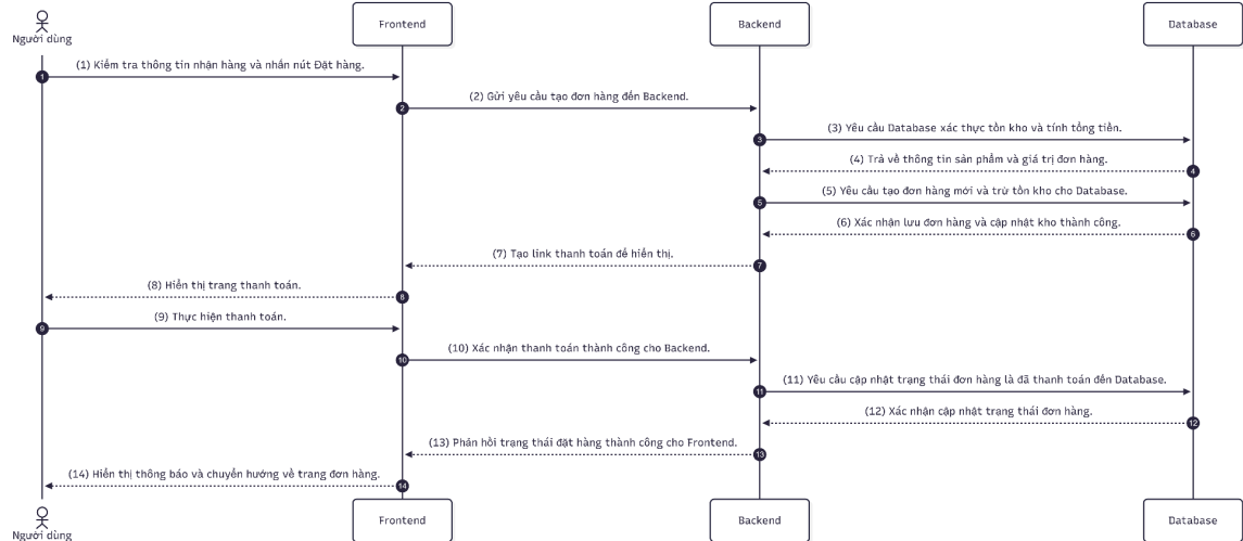
Hình 14 Sequence đặt hàng
