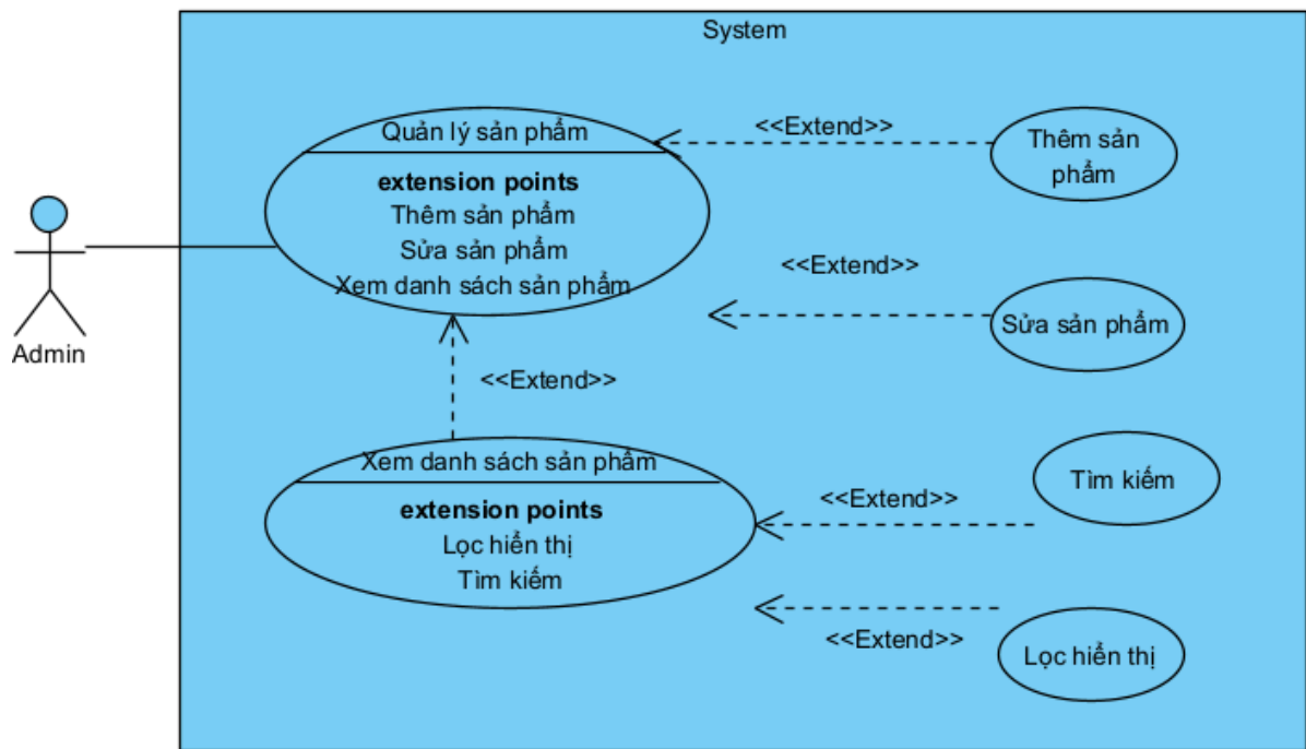
Hình 5 Use case quản lý sản phẩm
