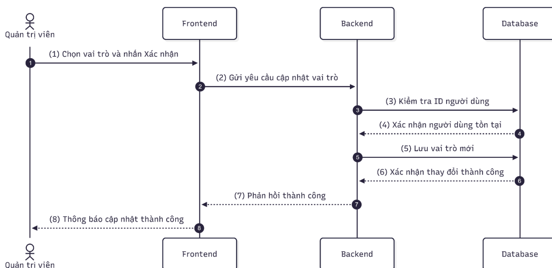
Hình 19 Sequence sửa vai trò user
