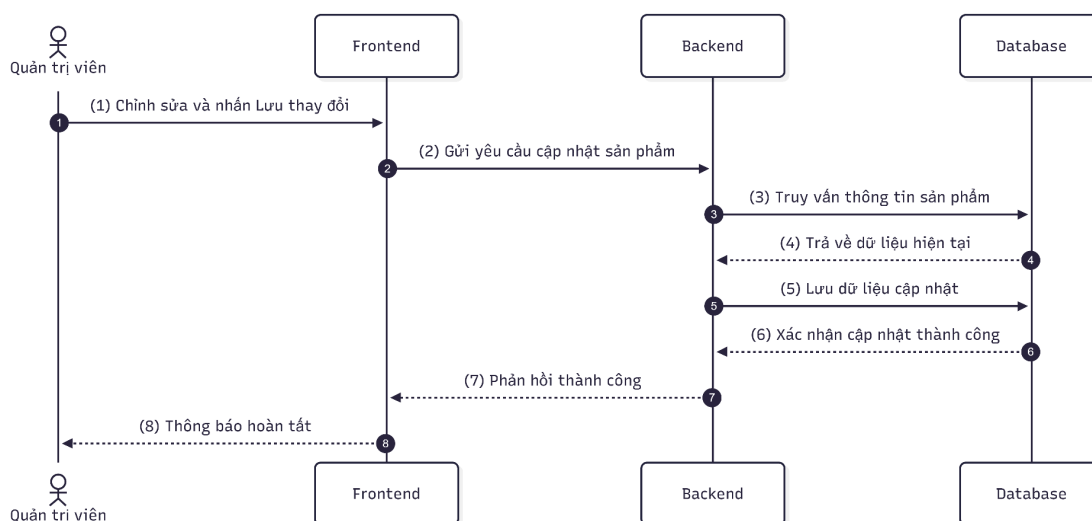
Hình 18 Sequence chỉnh sửa sản phẩm
