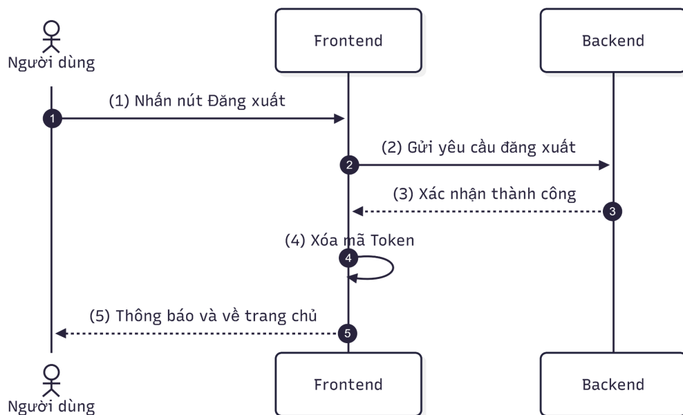
Hình 9 Sequence Đăng xuất
