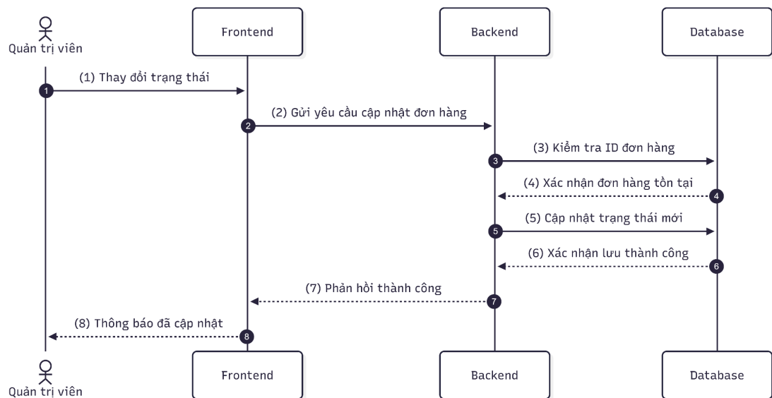
Hình 17 Sequence quản lý đơn hàng
